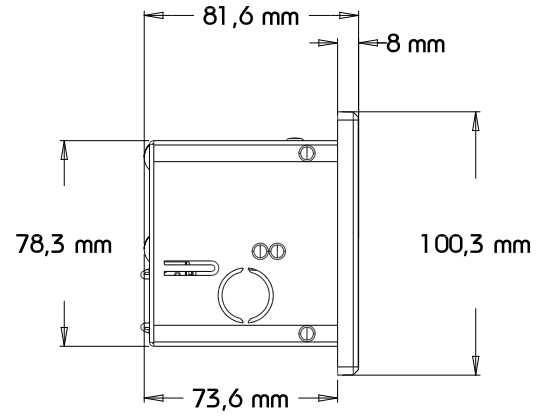
Ansicht Seite (links)
