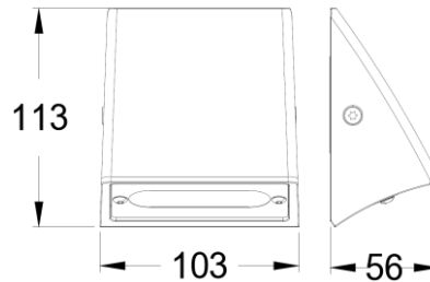
Maßzeichnung (Angaben in mm)
