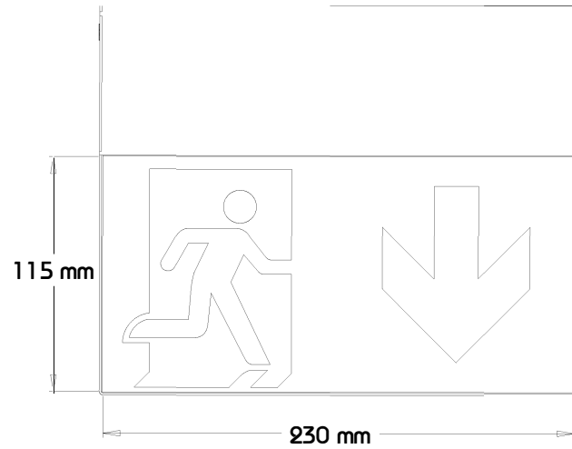
Ansicht Oben
