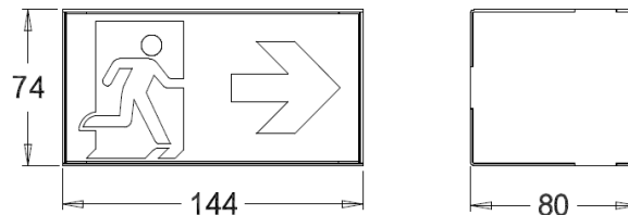
Maßzeichnung (Angaben in mm)
