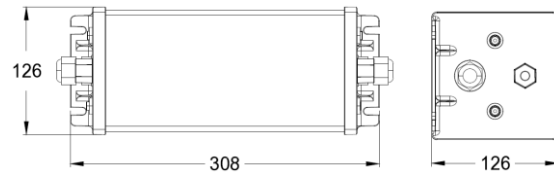
Maßzeichnung (Angaben in mm)
