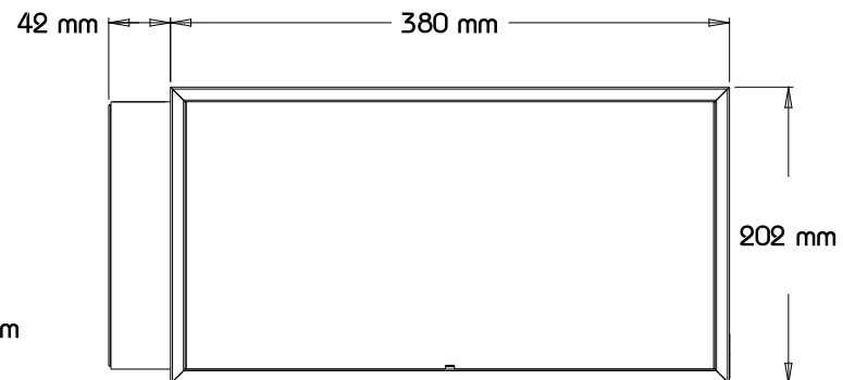
Ansicht Hinten
