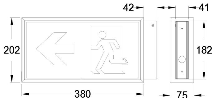
Maßzeichnung (Angaben in mm)
