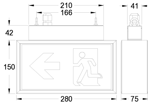
Maßzeichnung (Angaben in mm)
