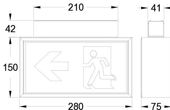
Maßzeichnung (Angaben in mm)
