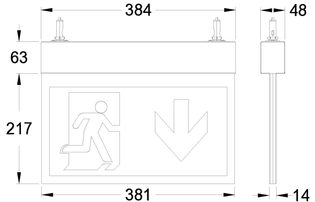
Maßzeichnung (Angaben in mm)
