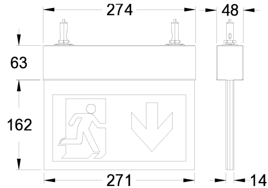
Maßzeichnung (Angaben in mm)
