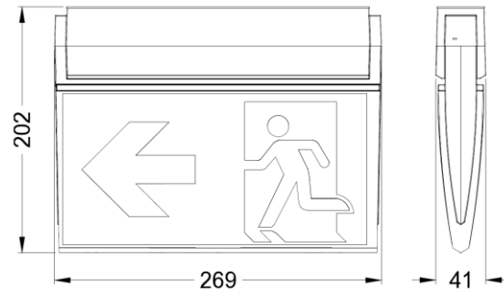
Maßzeichnung (Angaben in mm)
